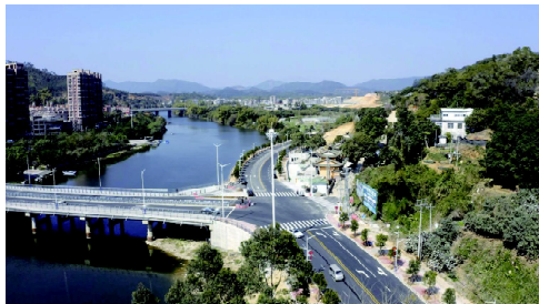
改造后的云漳大桥
