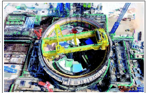
漳州核电1号机组反应堆压力容器吊装成功
